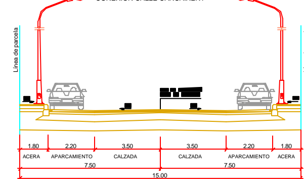
SECCION E-E SECCION CALLES TRANSVERSALES CONEXION CALLE CARCAIXENT
