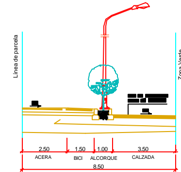
SECCION A-A SEMISECCION EL RODALET LADO OESTE SIN APARCAMIENTO
