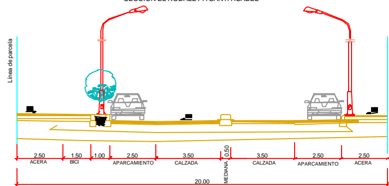
SECCION H-H SECCION EL RODALET A SANTA ISABEL
