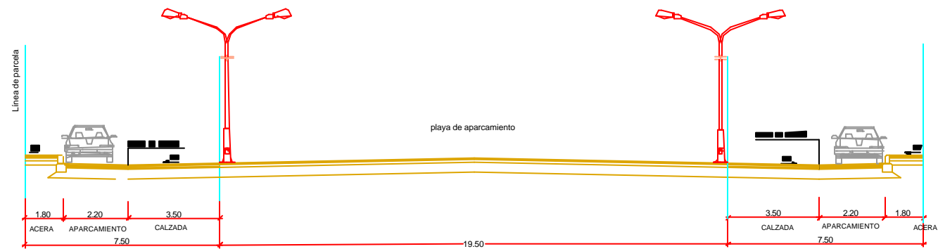
SECCION D-D SEMISECCION BULEVAR CENTRAL
