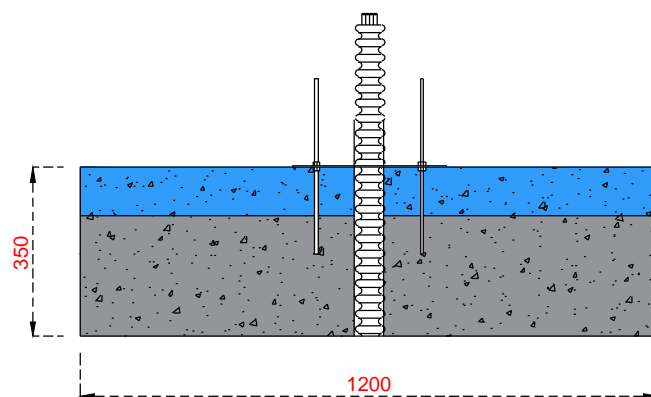
1 PEANA DE ANCLAJE - ALZADO ESCALA N/A @ A3
