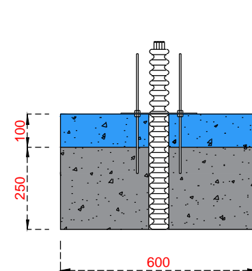
2 PEANA ANCLAJE - PERFIL LATERAL ESCALA N/A @ A3
